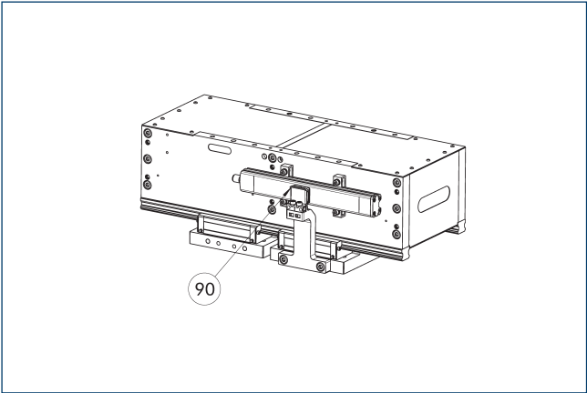
90 유도 위치 측정 시스템 "유도 위치 측정 시스템" 옵션을 통해 그리퍼의 전체 스트로크를 아날로그 수단으로 쿼리할 수 있습니다.
