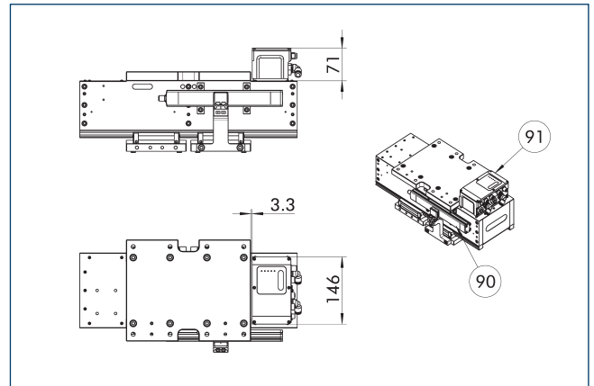
90 공압 포지셔닝 장치 PPD
