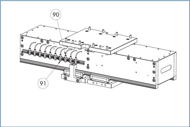
90 유도성 근접 스위치 91 부착 키트(유도성 근접 스위치용 홀더 포함)
