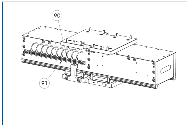
90 Indukcyjny czujnik zbliżeniowy 91 Zestaw montażowy łącznie z uchwytem indukcyjnego czujnika zbliżeniowego
