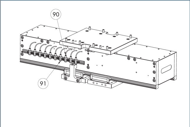
90 Индуктивный бесконтактный выключатель 91 Комплект подключения, в том числе крепление для индуктивного бесконтактного выключателя
