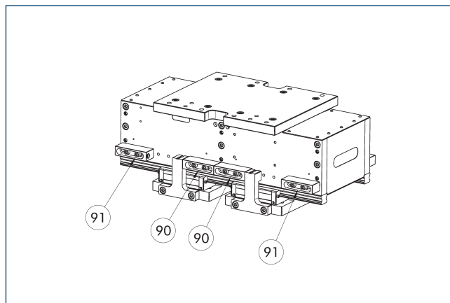
90 Ограничение хода в направлении закрытия
