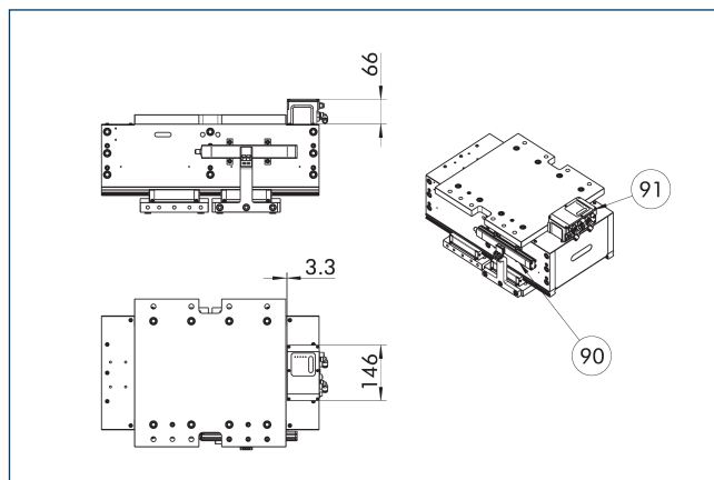
90 Пневматическое позиционирующее устройство PPD
