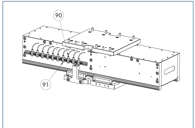
90 Inductieve naderingsschakelaar.
