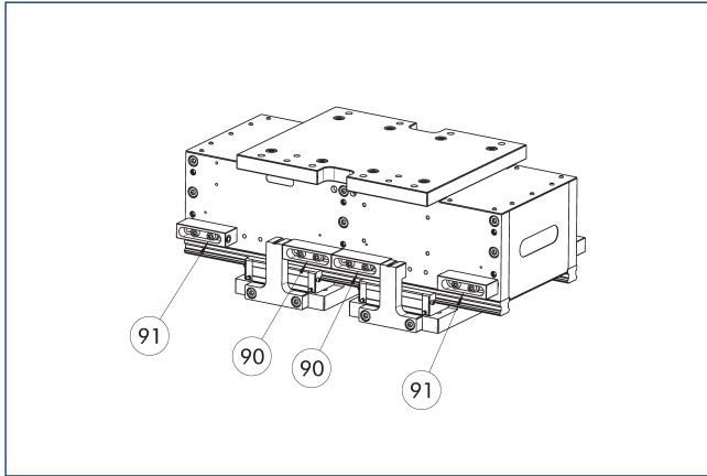
⑨⑩ 폐쇄 방향의 스트로크 제한
