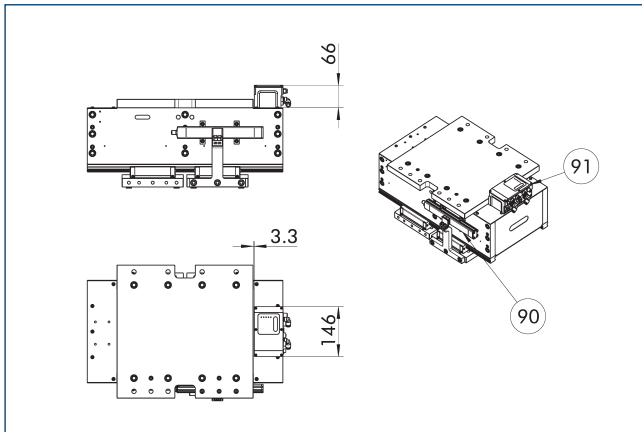
⑨⑩ 공압 포지셔닝 장치 PPD
