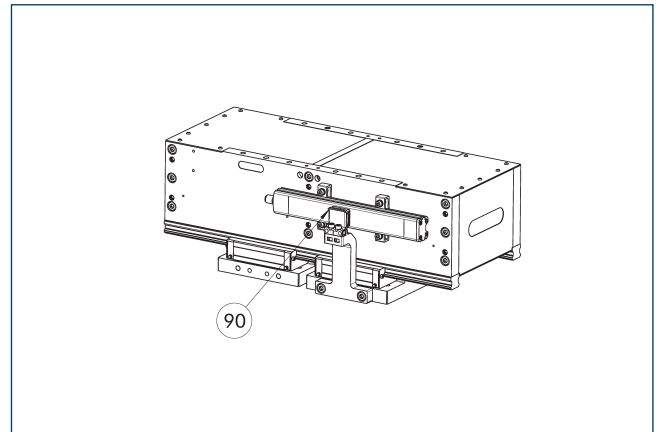
⑨⑩ 유도 위치 측정 시스템
