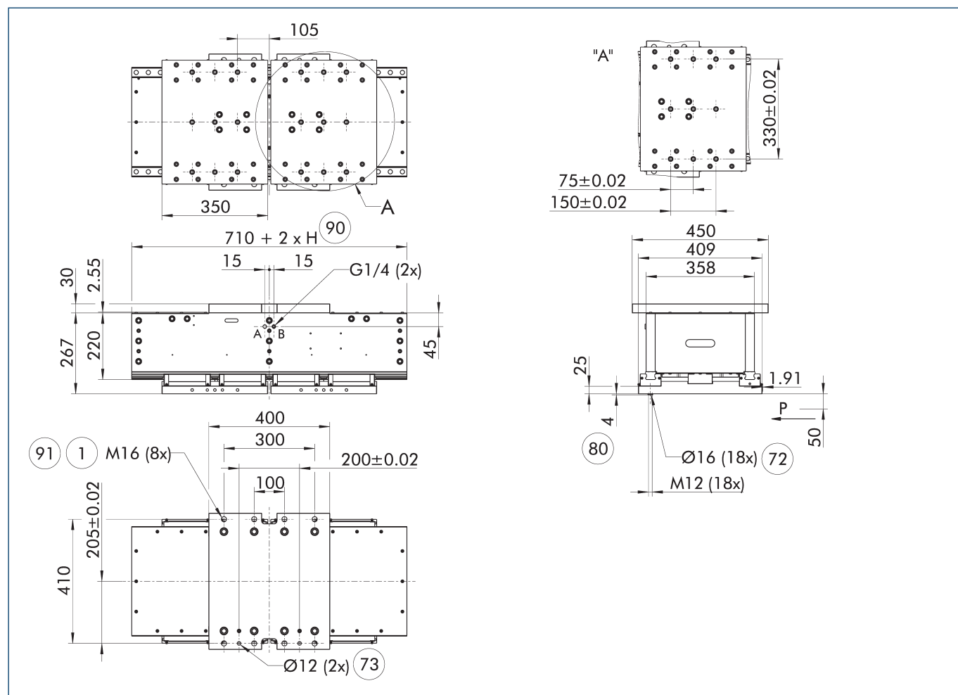
主视图 PLG 120-...-2-...
