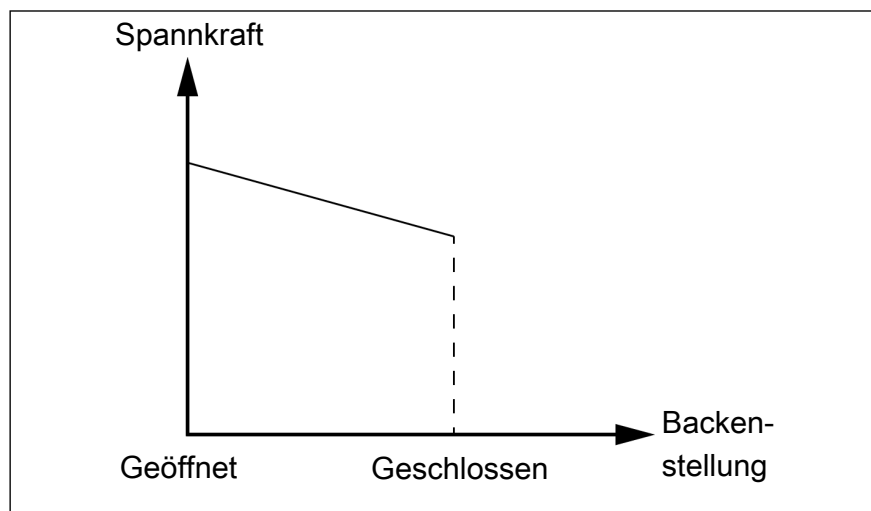
Abhängigkeit Spannkraft – Backenhub
