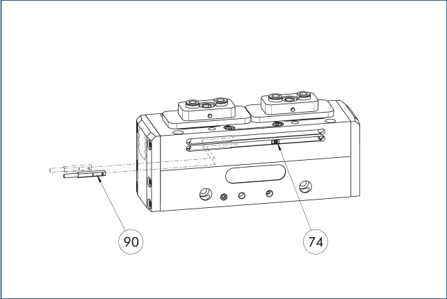
74 센서의 한계 정지 90 MMS 22-...-PI2-... 센서
