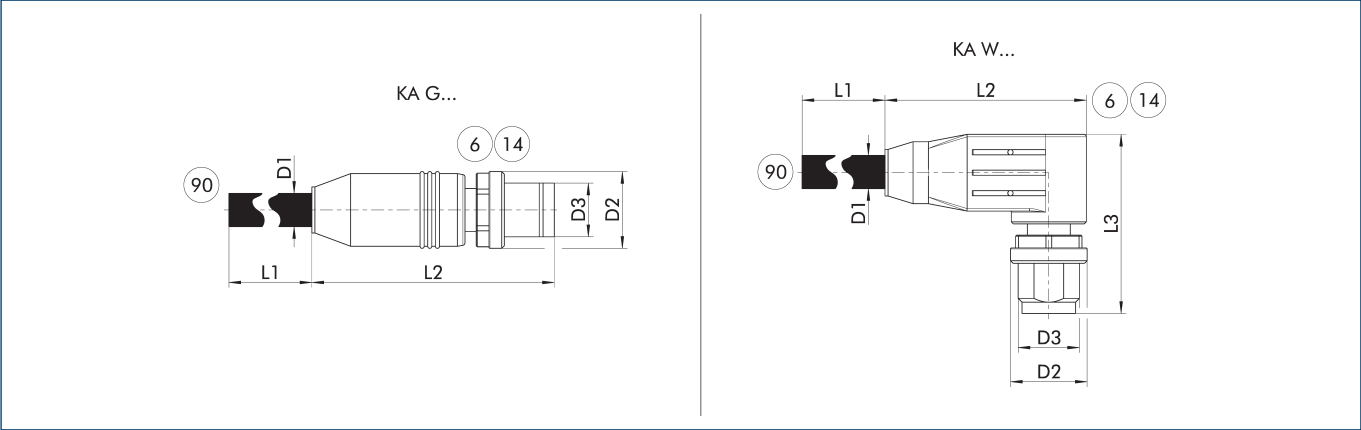
KA G...Rechte connectoraansluiting KA W...Haakse connectoraansluiting 6Aansluiting modulezijde 14Connector 90Kabeluiteinden met tweede connectoraansluiting
