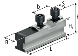
SFG Grundbacken
