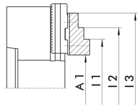
Grundbackenstellung II
