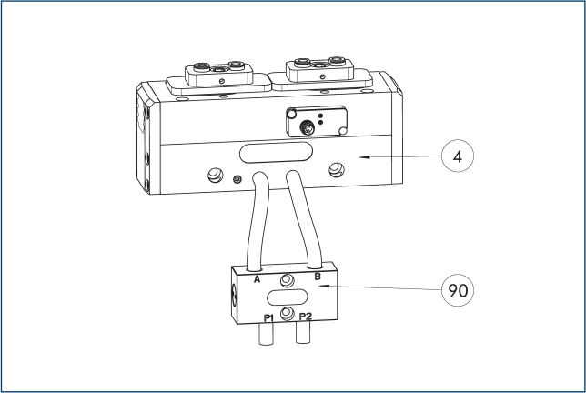
❶ Захваты ❾ Клапан поддержания давления SDV-P
