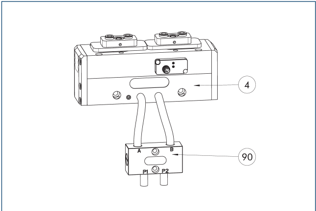
❶ Захваты ❾❶ Клапан поддержания давления SDV-P
