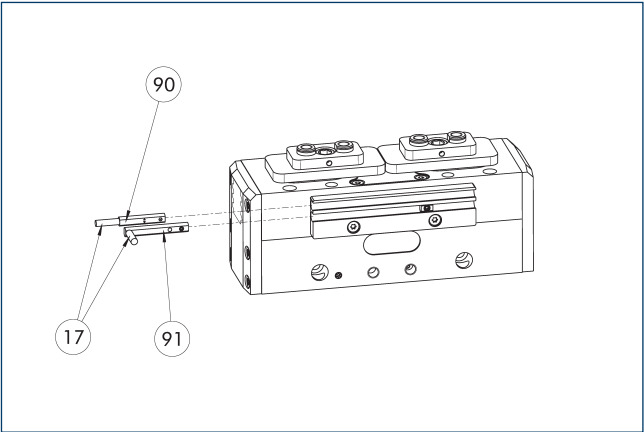
①7 ケーブルアウトレット ⑨1 センサー MMS 22 ..-PI1-...-SA ⑨0 センサー MMS 22 PI1-...
