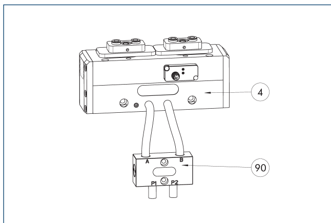
⑨0 SDV-P klep voor drukbehoud
