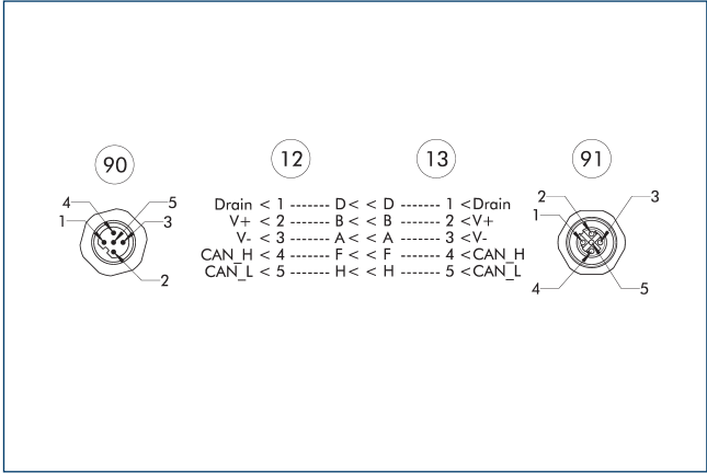
12 Ведущая сторона 90 Разъем M12, кодировка A 13 Переходная сторона 91 Гнездо M12, маркировка A
