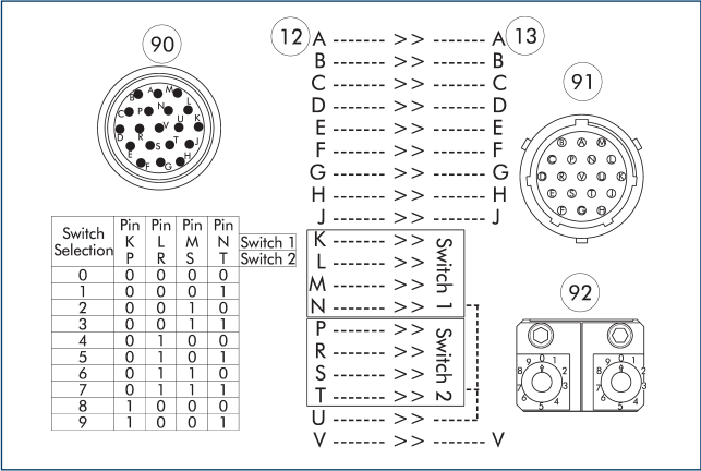
Расположение контактов для SWO-S19-K и SWO-S10-A
