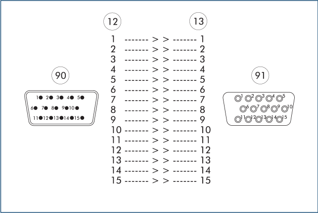
12 Ведущая сторона 90 Разъем D-sub 13 Переходная сторона 91 Штекер D-sub
