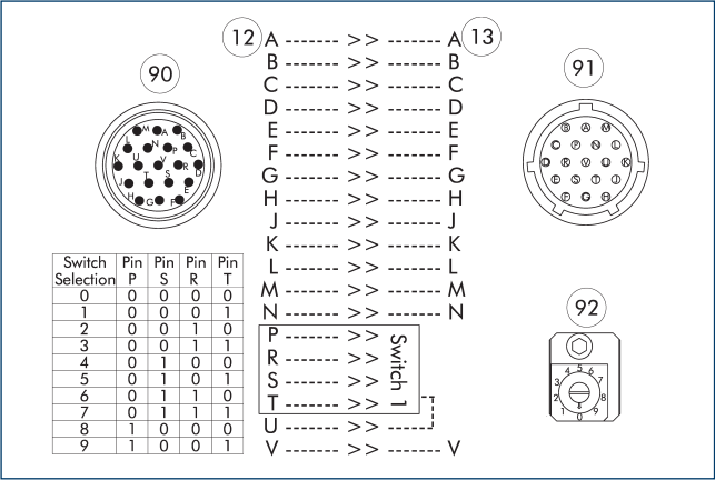
Расположение контактов для SWO-S19-K и SWO-S14-A
