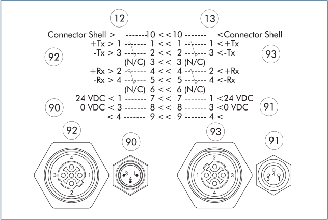
12 Ведущая сторона 13 Переходная сторона 90 Разъем M8, кодировка A, 3 контакта 91 Гнездо M8, маркировка A, 3 контакта 92 Гнездо M12 с ключом «D» 93 Гнездо M12 с ключом «D»
