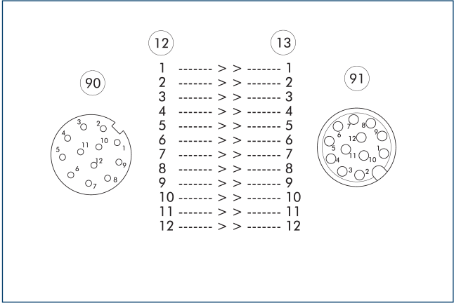
12 Ведущая сторона 90 Разъем M12, кодировка A, 12 контактов 13 Переходная сторона 91 Гнездо M12, маркировка A, 12 контактов
