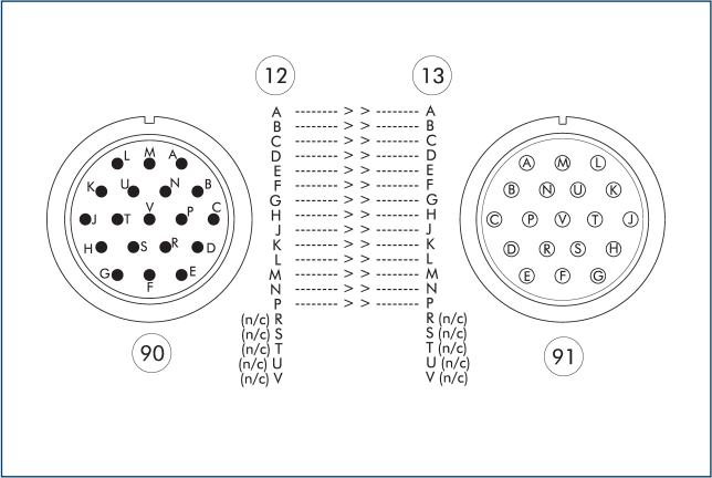
12 Ведущая сторона 13 Переходная сторона 90 Разъем Amphenol MS с резьбовым наконечником, 19 контактов 91 Гнездо Amphenol MS с резьбовым наконечником, 19 контактов
