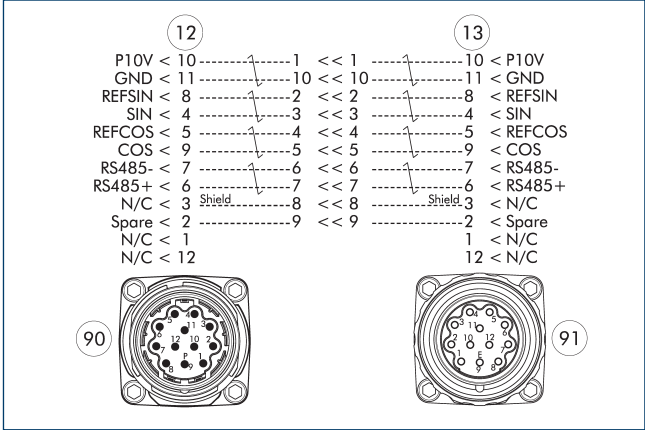
12 Ведущая сторона 90 Разъем M23, 12 контактов 13 Переходная сторона 91 Гнездо M23, 12 контактов
