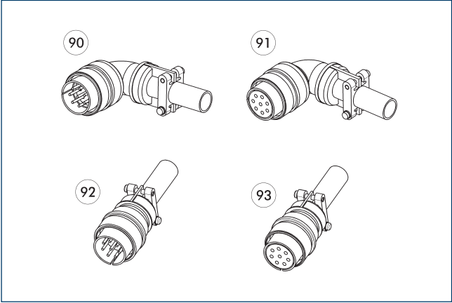
90 Угловой штекер 92 Прямой штекер 91 Угловое гнездо 93 Прямое гнездо
