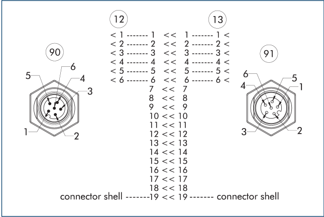
12 Ведущая сторона 90 Разъем M12, кодировка A, 6 контактов 13 Переходная сторона 91 Гнездо M12, маркировка A, 6 контактов
