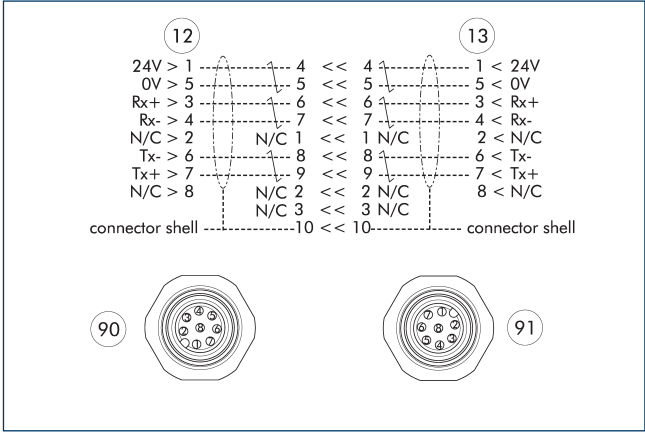
12 Ведущая сторона 90 Гнездо M12, маркировка A, 8 контактов 13 Переходная сторона 91 Разъем M12, кодировка A, 8 контактов
