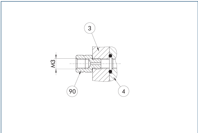
3 Adaptador 90 Estrangulador fijo 4 Unidad de giro
