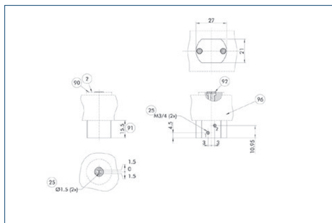
2 Collegamento della struttura
