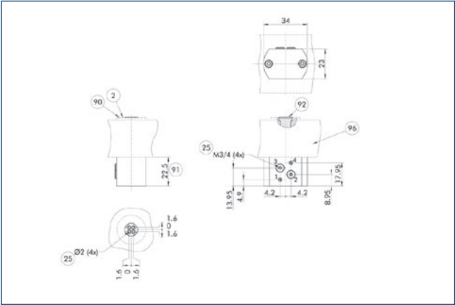
2 Collegamento della struttura 25 Tubazione fluido 90 Il piano di fissaggio può essere desunto dal disegno dell'unità di base 91 Dimensioni aggiuntive del modulo collegato, opzione MDF 92 Guarnizione 96 Base SRM
