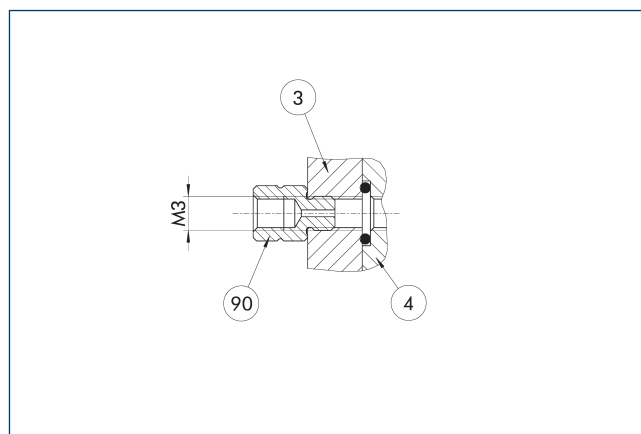
3 Piastra adattatrice
