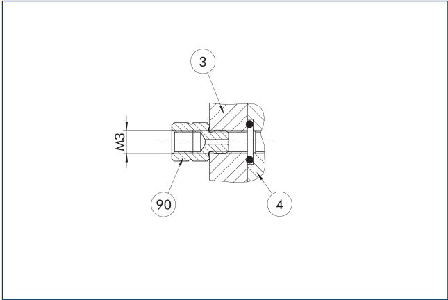
3 Piastra adattatrice 90 Valvola a farfalla fissa 4 Attuatore rotante
