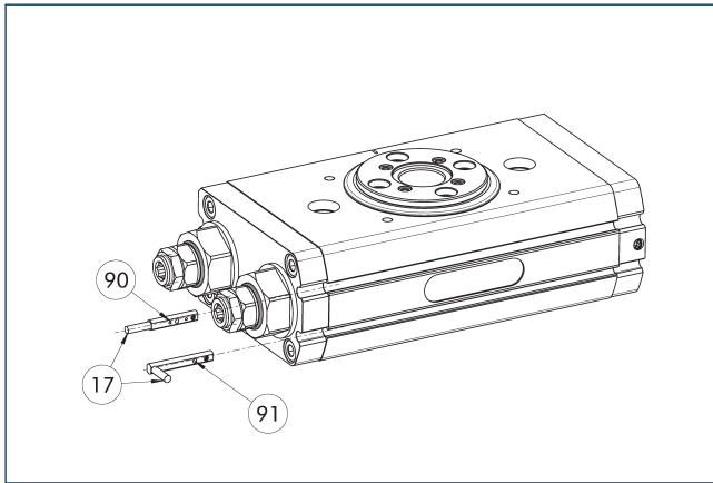
① 케이블 콘센트 ⑨ 센서 MMS 22-...-SA ⑨ 센서 MMS 22-...
