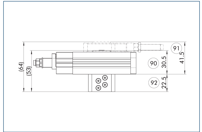
90 SRM 기본 버전 총 높이 (댐핑 방식 H/E 유형) 92 부착된 모듈의 추가 치수, 옵션 MDF
