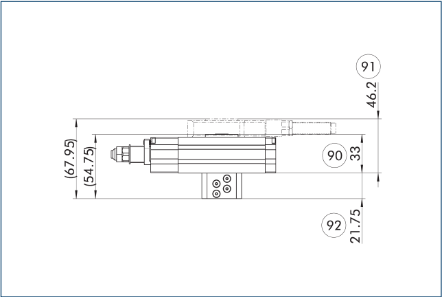
90 SRM 기본 버전 총 높이(댐핑 방식 H/E/S)
