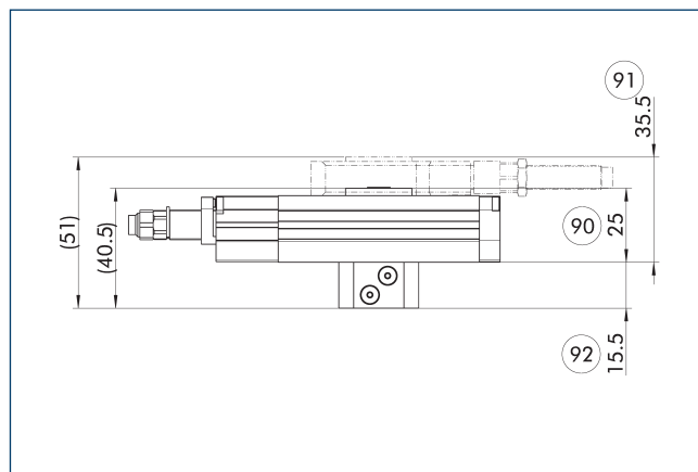
90 SRM 기본 버전 총 높이 (댐핑 방식 H/E 유형)
