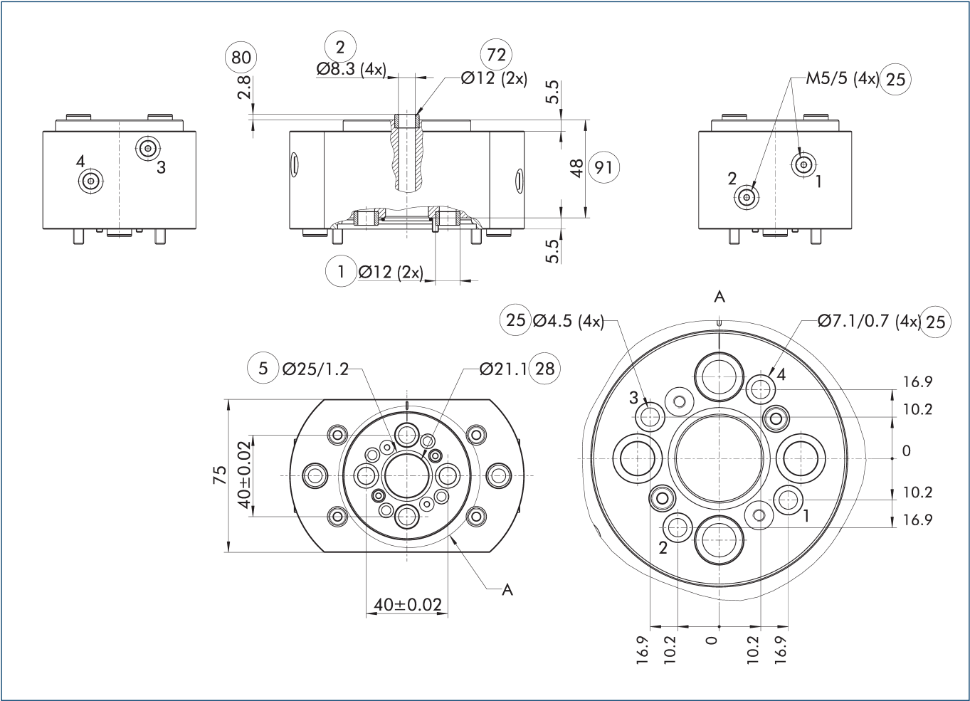
図面はベースモジュールおよびその他の旋回ユニット 用オプションなしの、メディアフィードスルーのオプションを示します。
