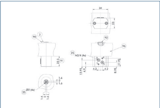
2 Collegamento della struttura 91 Dimensioni aggiuntive del modulo collegato, opzione MDF 25 Tubazione fluido 92 Guarnizione 90 Il piano di fissaggio può essere desunto dal disegno dell'unità di base 96 Base SRM
