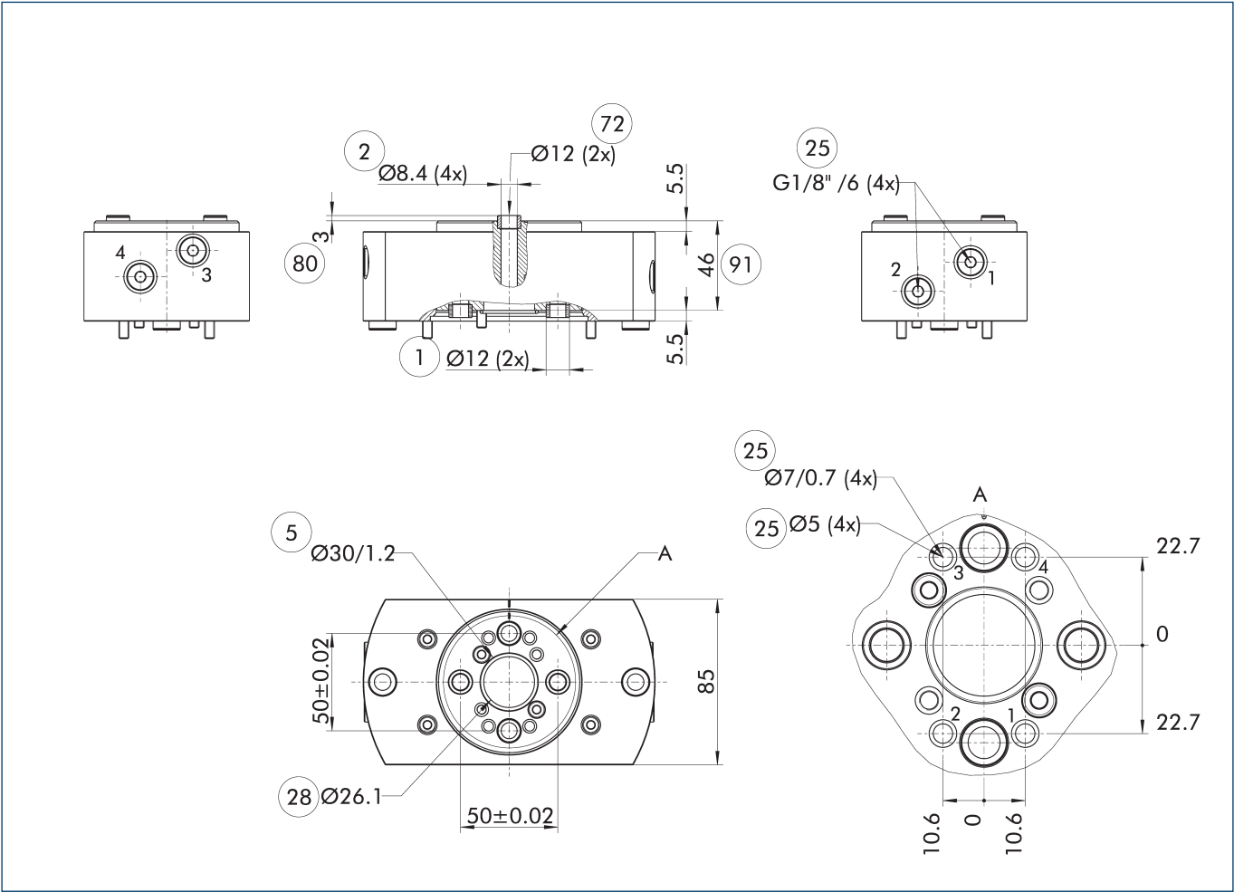
Le plan montre l'option joint tournant pneumatique, sans le module de base ni autres options de l'unité de rotation. 1 Fixation de l'unité de rotation 2 Fixation de la charge 5 Joint torique 25 Passages pneumatiques 28 Perçage 72 Ajustement pour douilles de centrage 80 Dépassement des douilles de centrage 91 Dimensions option MDF
