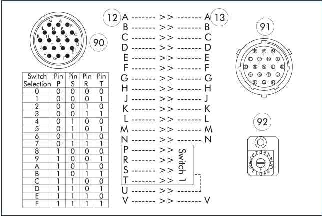
SWO-K19-K 与 SWO-K14-A 的针脚触点布局
