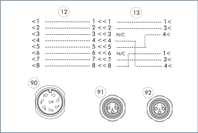
⑫ 主侧 ⑨① M8 插座, A 码, 3 针 ⑬ 转接头侧 ⑨② M8 插座, A 码, 3 针 ⑨⑩ M8 连接器, A 码, 8 针
