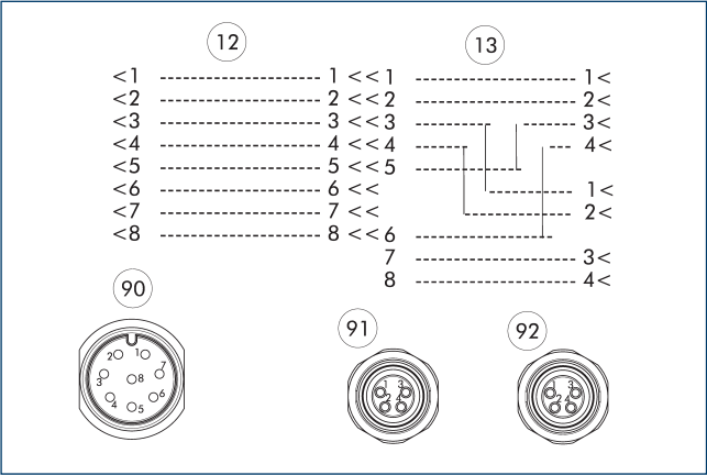
⑫ 主侧 ⑨① M8 插座, A 码, 4 针 ⑬ 转接头侧 ⑨② M8 插座, A 码, 4 针 ⑨⑩ M8 连接器, A 码, 8 针
