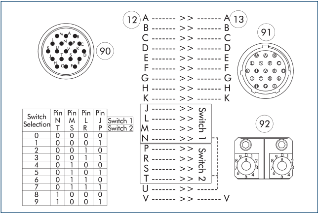
SWO-K19-K 与 SWO-K10-A 的针脚触点布局
