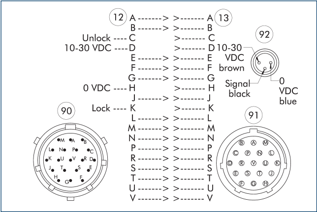
SWO-K19W-K 和 SWO-K19-A 的引脚分配
