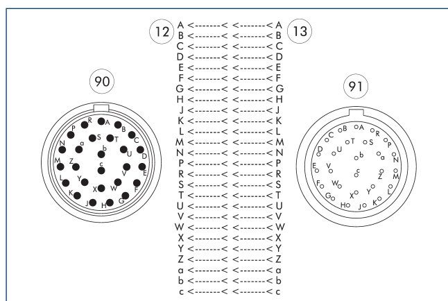
⑨⑩ Amphenol PT バヨネットロック コネクタ, 26 ピン
