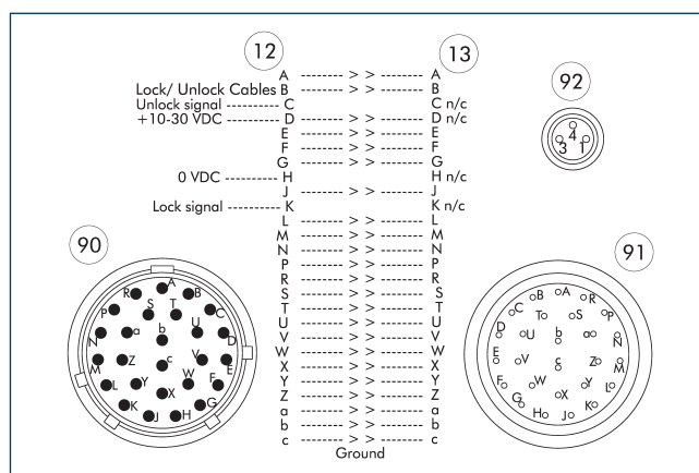
⑨1 Amphenol PT バヨネットロック ソケット, 26 ピン
