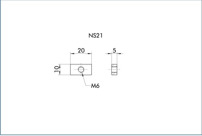
装置可以用 T 形螺母固定到位。精确的安装位置在相邻连接图上标明。
