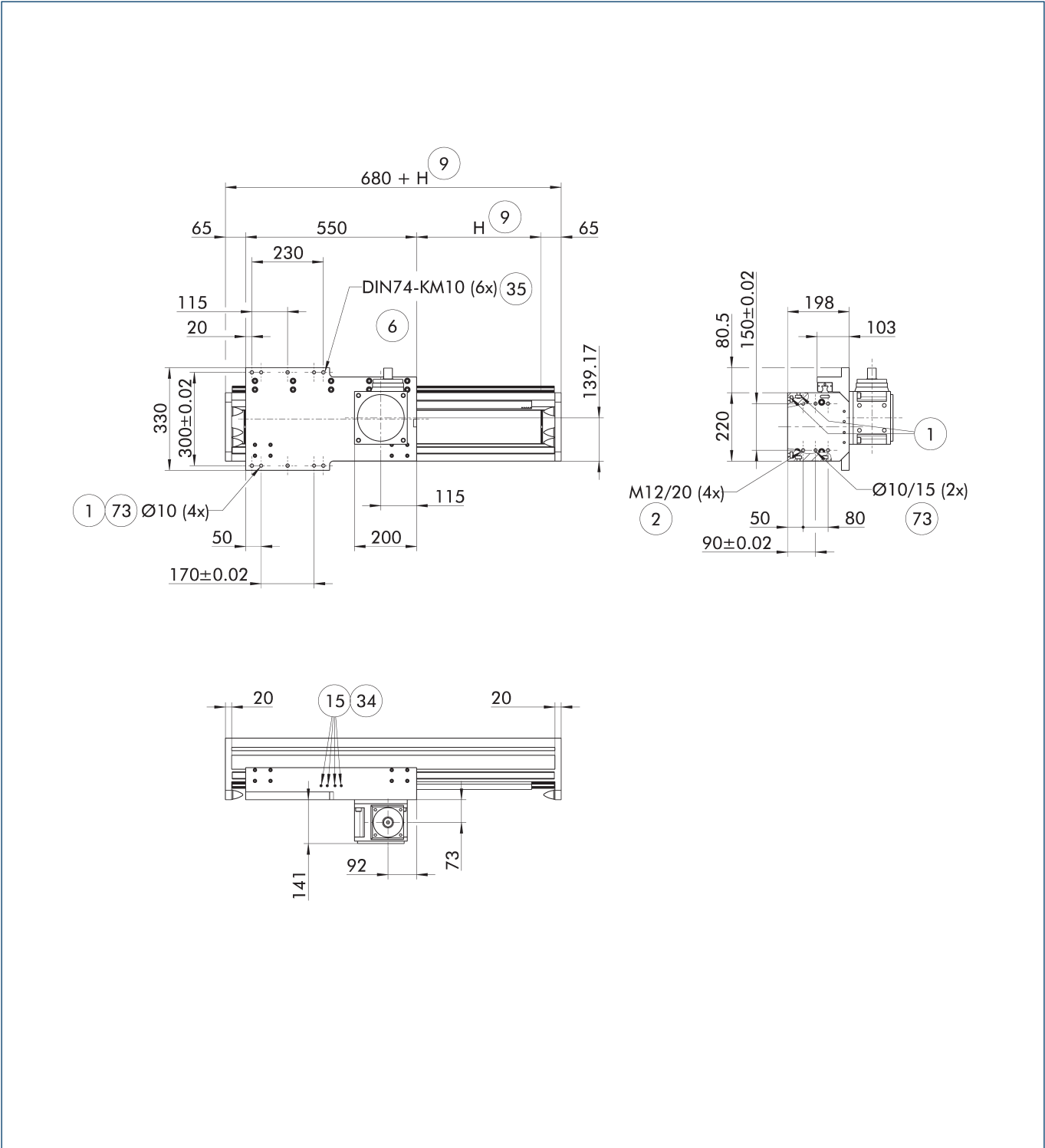
主视图 AZSH-M2
