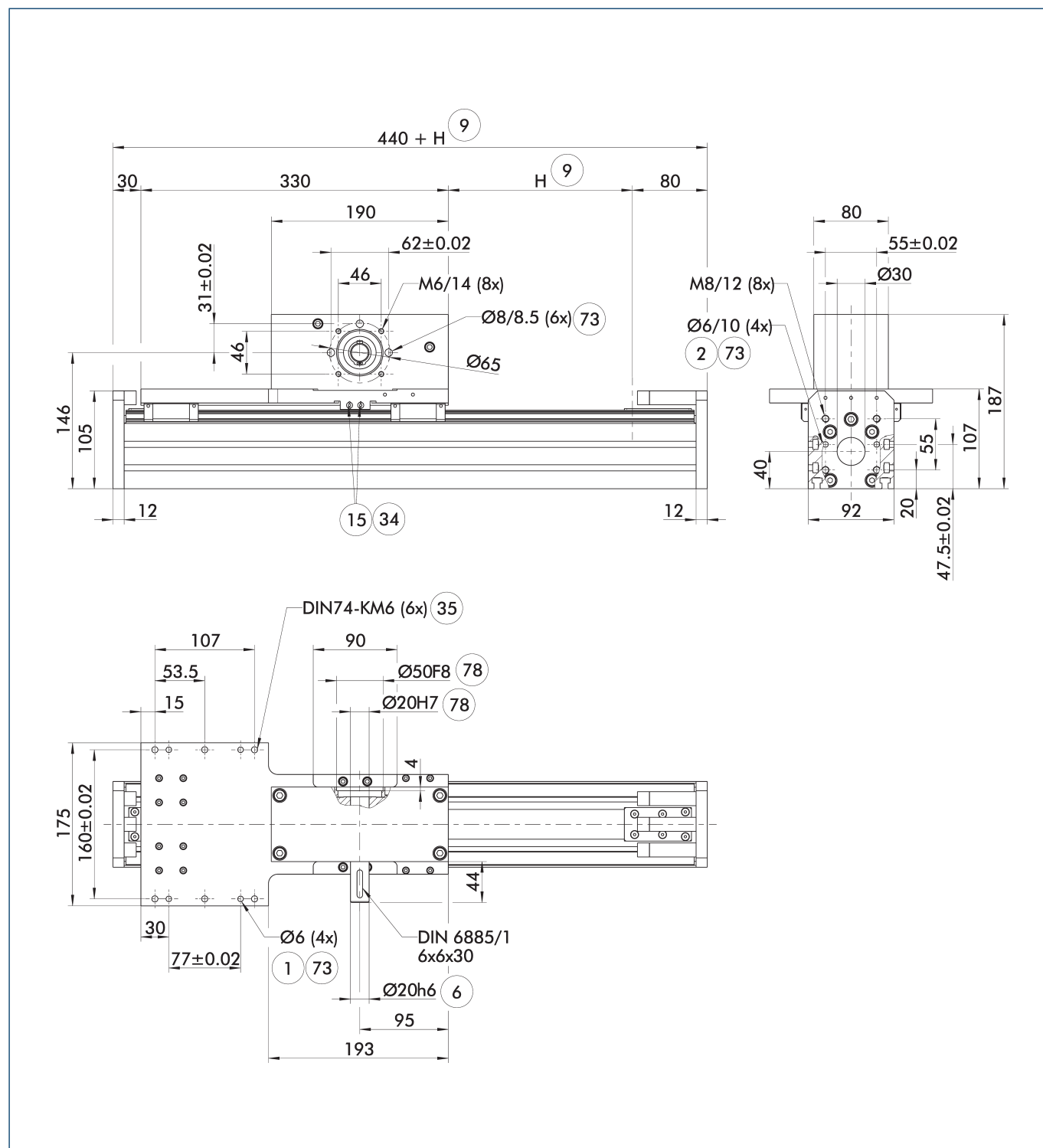
ASH 主视图
