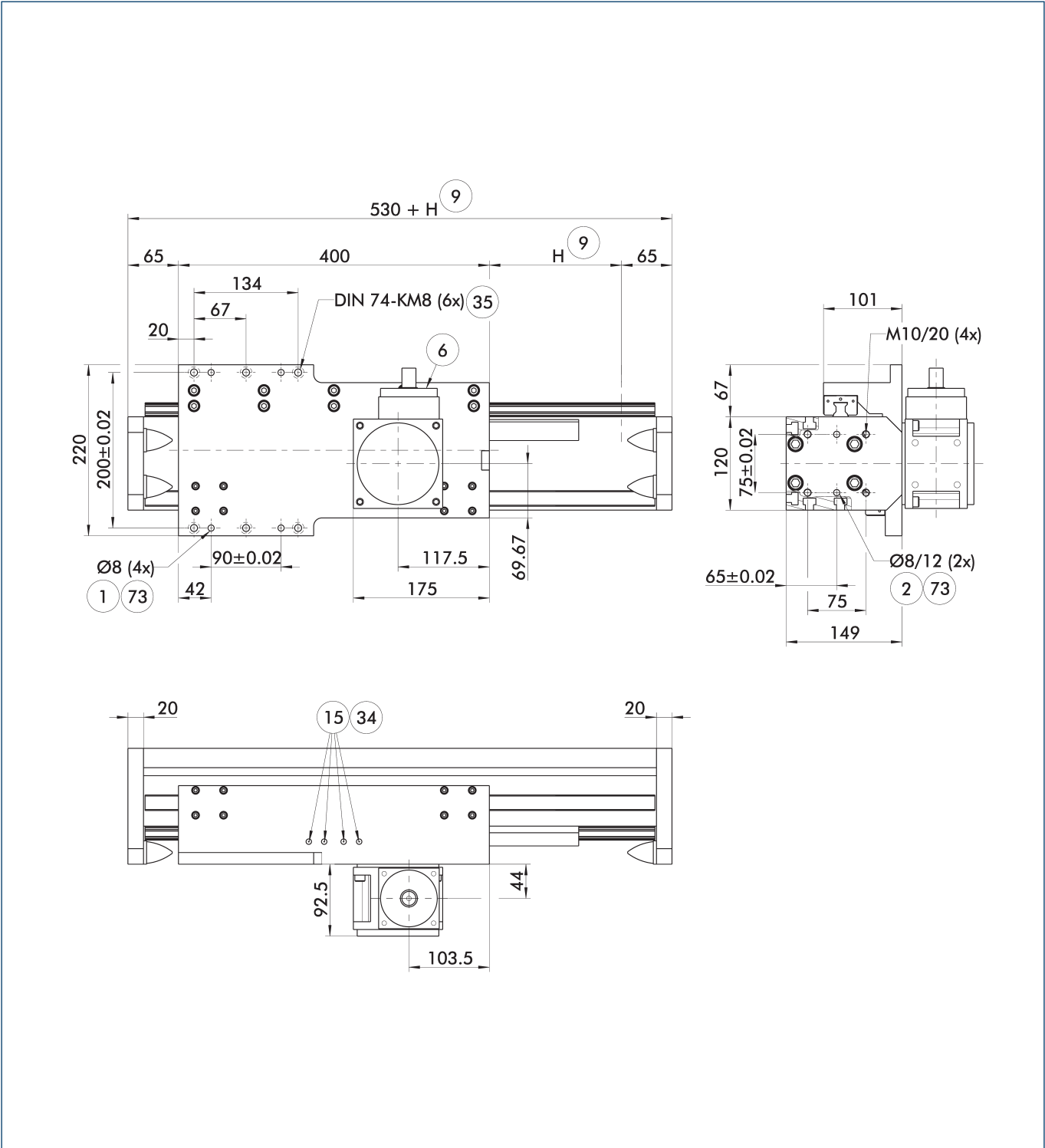
AZSH 主视图
