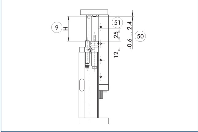
9 有效行程 50 阻尼行程调整范围 此图显示出可能的缩回位置微调。
