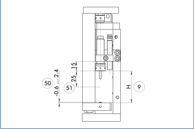
9 有效行程 50 阻尼行程调整范围 此图显示出可能的伸出位置微调。
