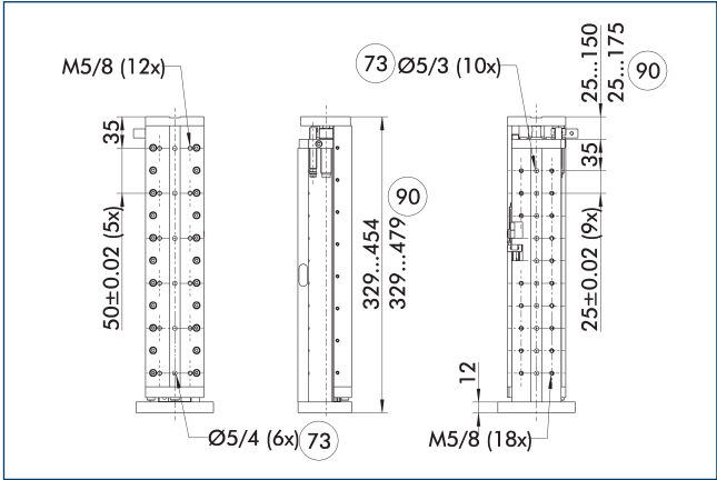
73 适合定心销 90 适用行程型号 H150 并非所有尺寸均标注在主视图上。
