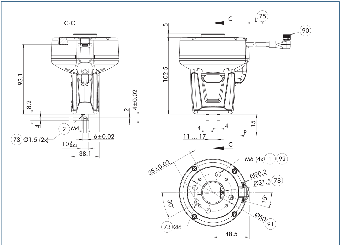
主视图 Co-act EGP-C 25-N-N-URID
