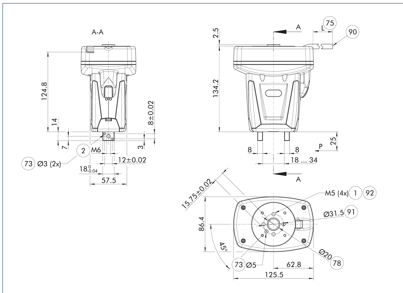
主视图 Co-act EGP-C 50-N-N-FCR7
