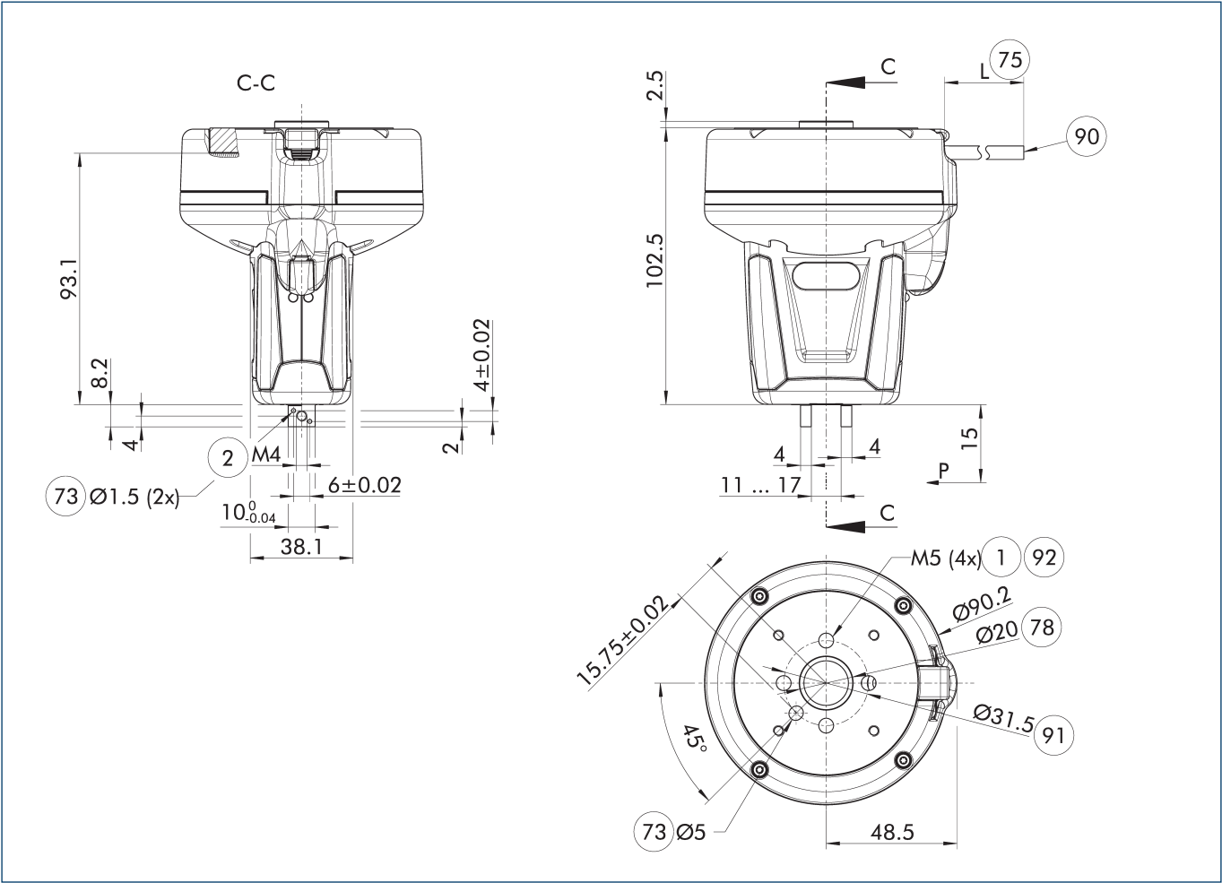
主视图 Co-act EGP-C 25-N-N-FCR7
