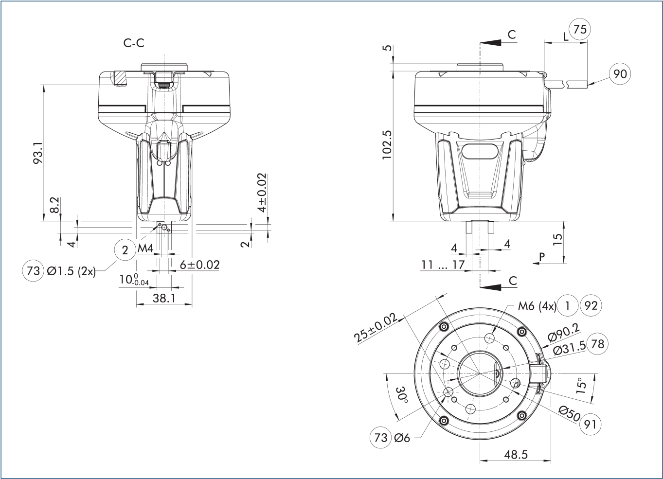
主视图 Co-act EGP-C 25-N-N-UREK
