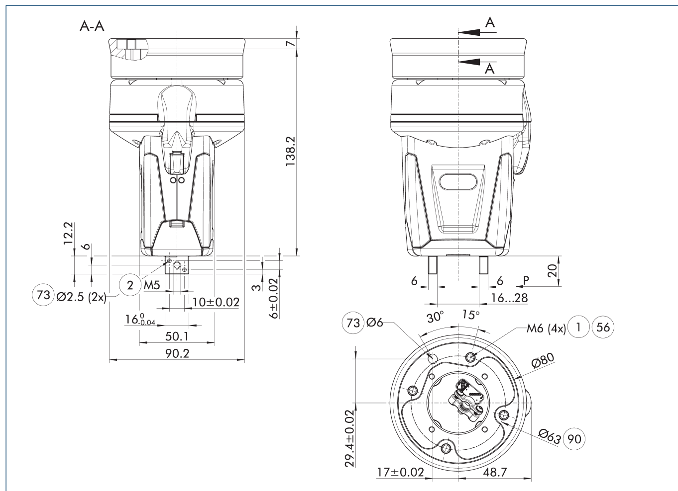
主视图 Co-act EGP-C 40 N-N-YHCP
