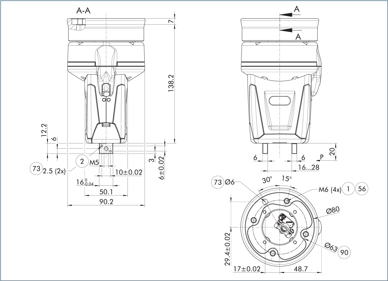
主视图 Co-act EGP-C 40 N-N-YHCN
