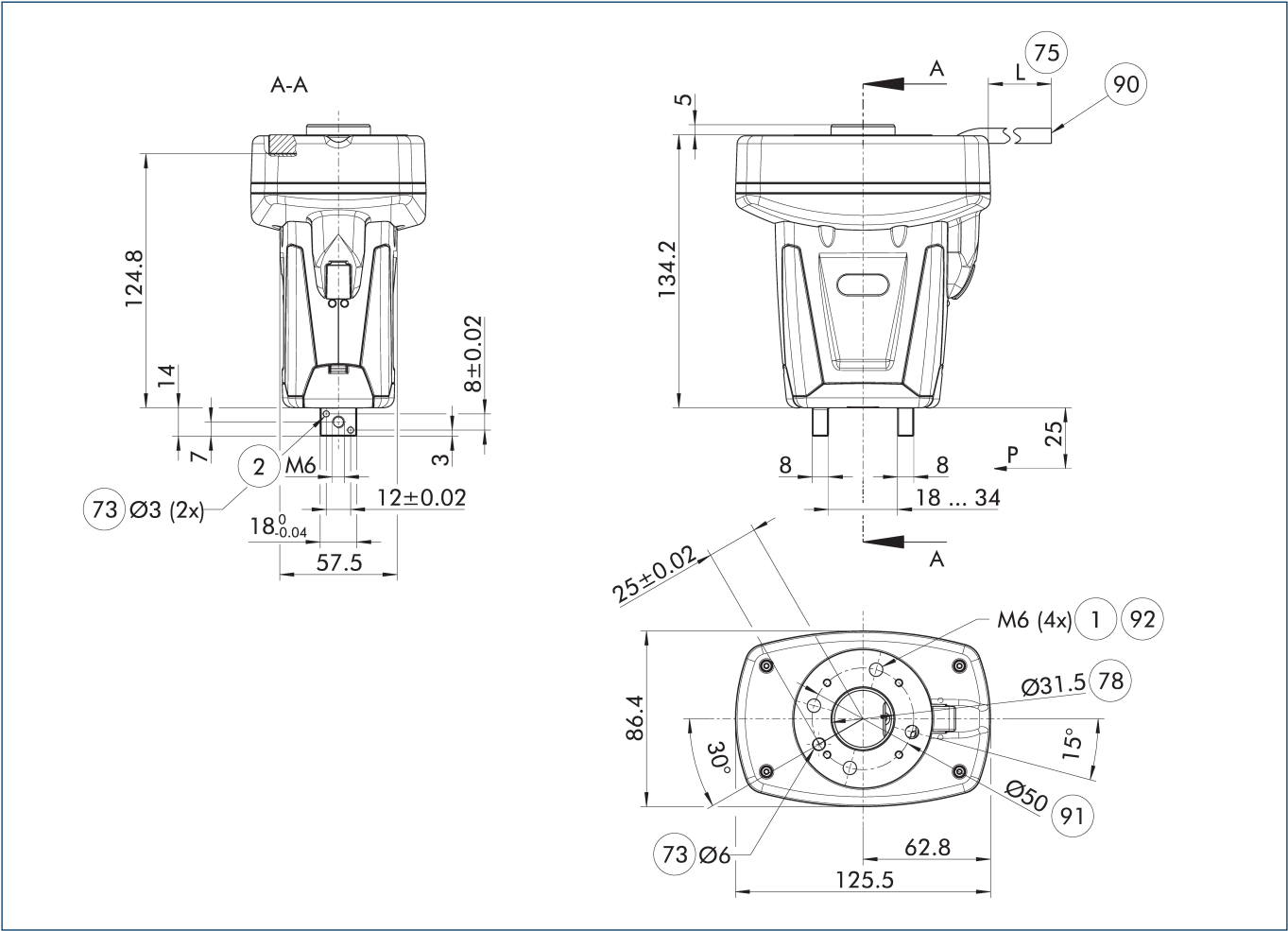
主视图 Co-act EGP-C 50-N-N-UREK
