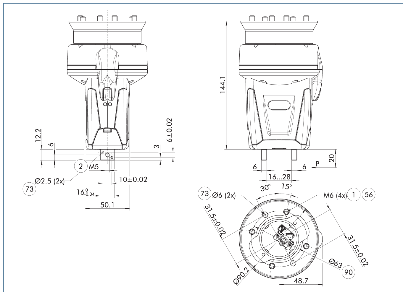
主视图 Co-act EGP-C 40 N-N-YDTP
