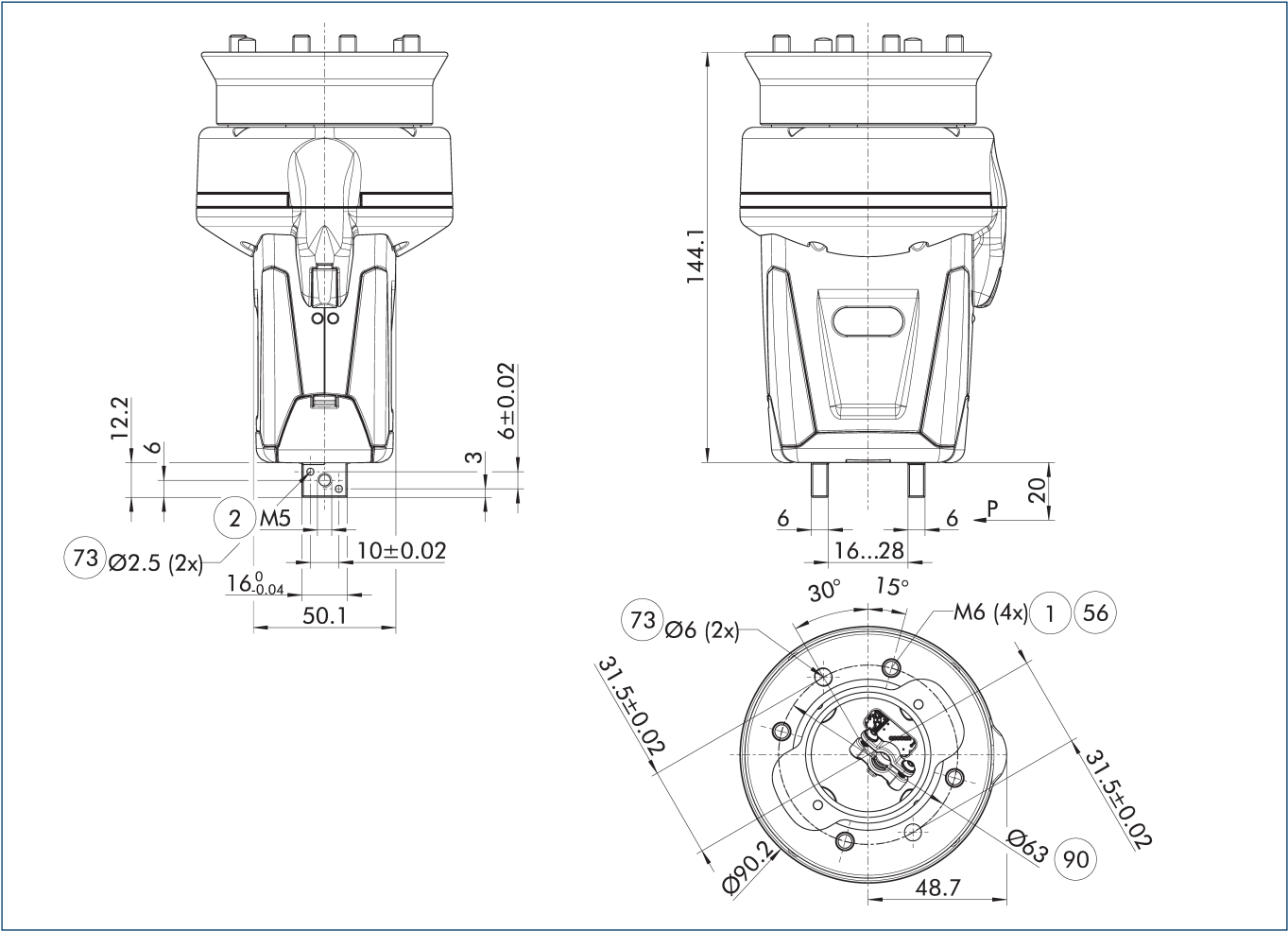
主视图 Co-act EGP-C 40 N-N-YDTN
