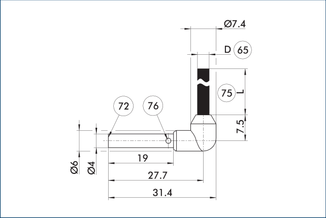
IN(K) 40-SA 主视图
