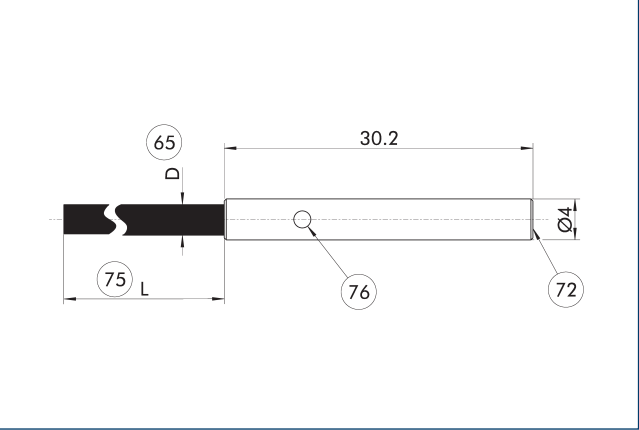
IN 40L 主视图
