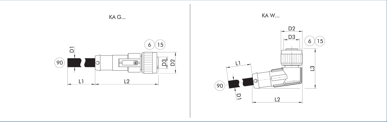
KA G... 带直插头连接器的连接电缆 KA W... 带角插头连接器的连接电缆 ⑥ 连接模块侧 ⑬ 插座 ⑨⑩ 电缆端带有明绞线
