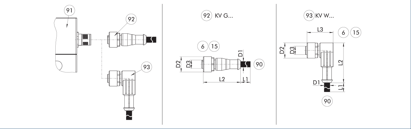
电缆延长线用于将相关组件连接到控制系统或用作延长电缆。延长线的模块侧配备一个 4 针 M8 插座（采用直式或弯式设计），而在另一侧配备一个 4 针 M8 连接器（直式）。电缆延长线可用于电缆槽和旋转应用。 ⑥ 连接模块侧 ⑬ 插座 ⑨⑩ 电缆端头，带直式连接器 ⑨⑩ 连接插头组件 ⑨⑩ 带直式母头连接器的电缆 ⑨⑩ 带角式母头连接器的电缆
