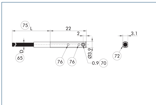
MMS(K) 22-PI2-HD 主视图
