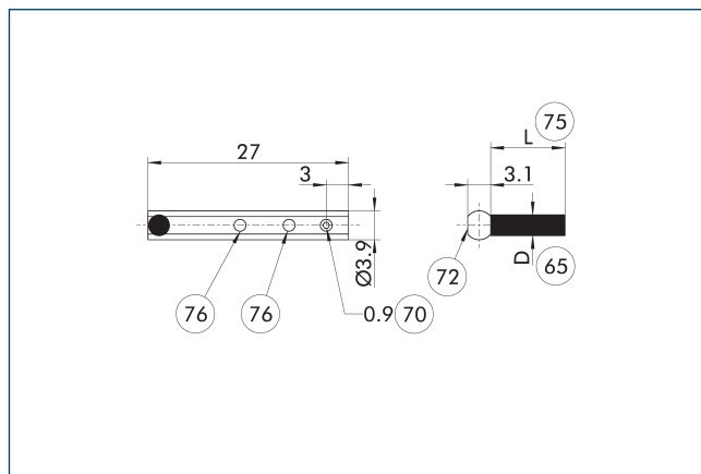
MMS(K) 22-PI2-SA 主视图
