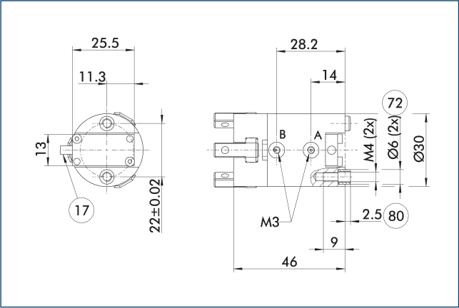
17 Кабельный выход 80 Глубина отверстия центрирующей втулки в ответной детали
