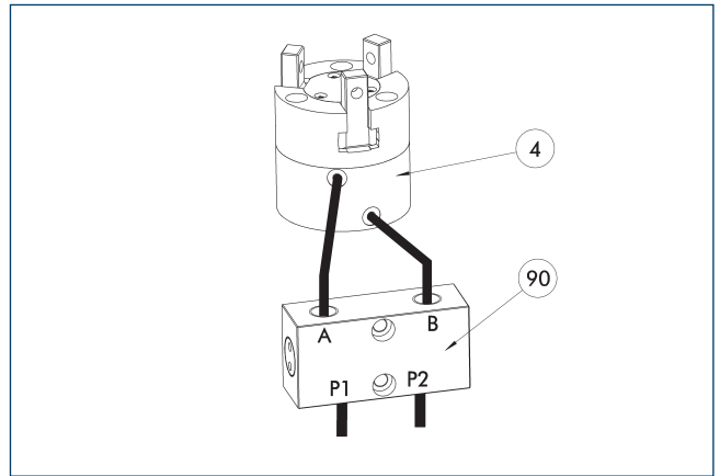
④ Uchopovače
