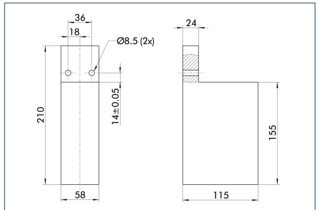
Výkres znázorňuje polotovar prsta, ktorý môže zákazník prepracovať.
