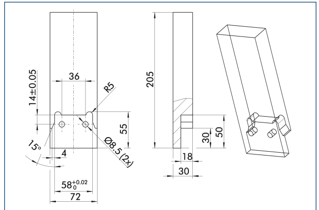
Návrh rozmerov pripojení prstov uchopovača
