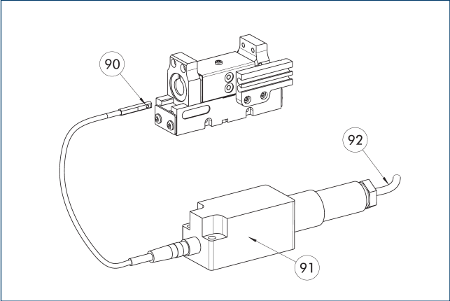
90 Snímač MMS 22-A-... 92 Připojovací kabely 91 Vyhodnocovací elektronika FPS-F5
