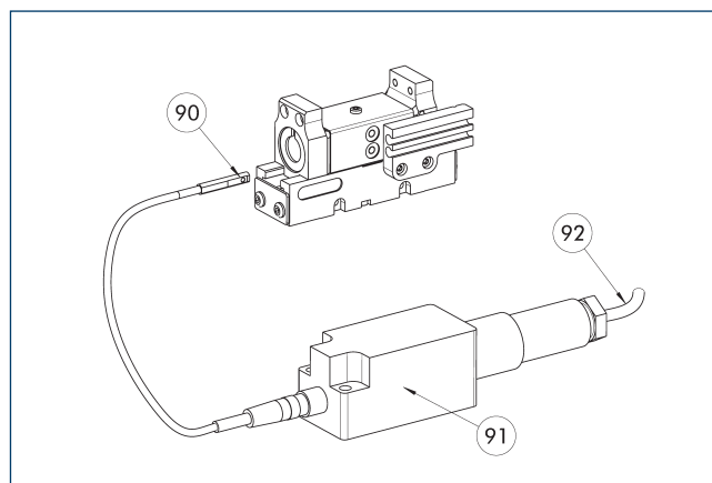
90 Датчик MMS 22-A-... 92 Соединительные кабели 91 Анализирующая электроника FPS-F5
