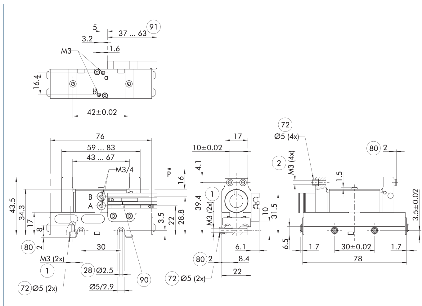
Главный вид KGG 70-24
