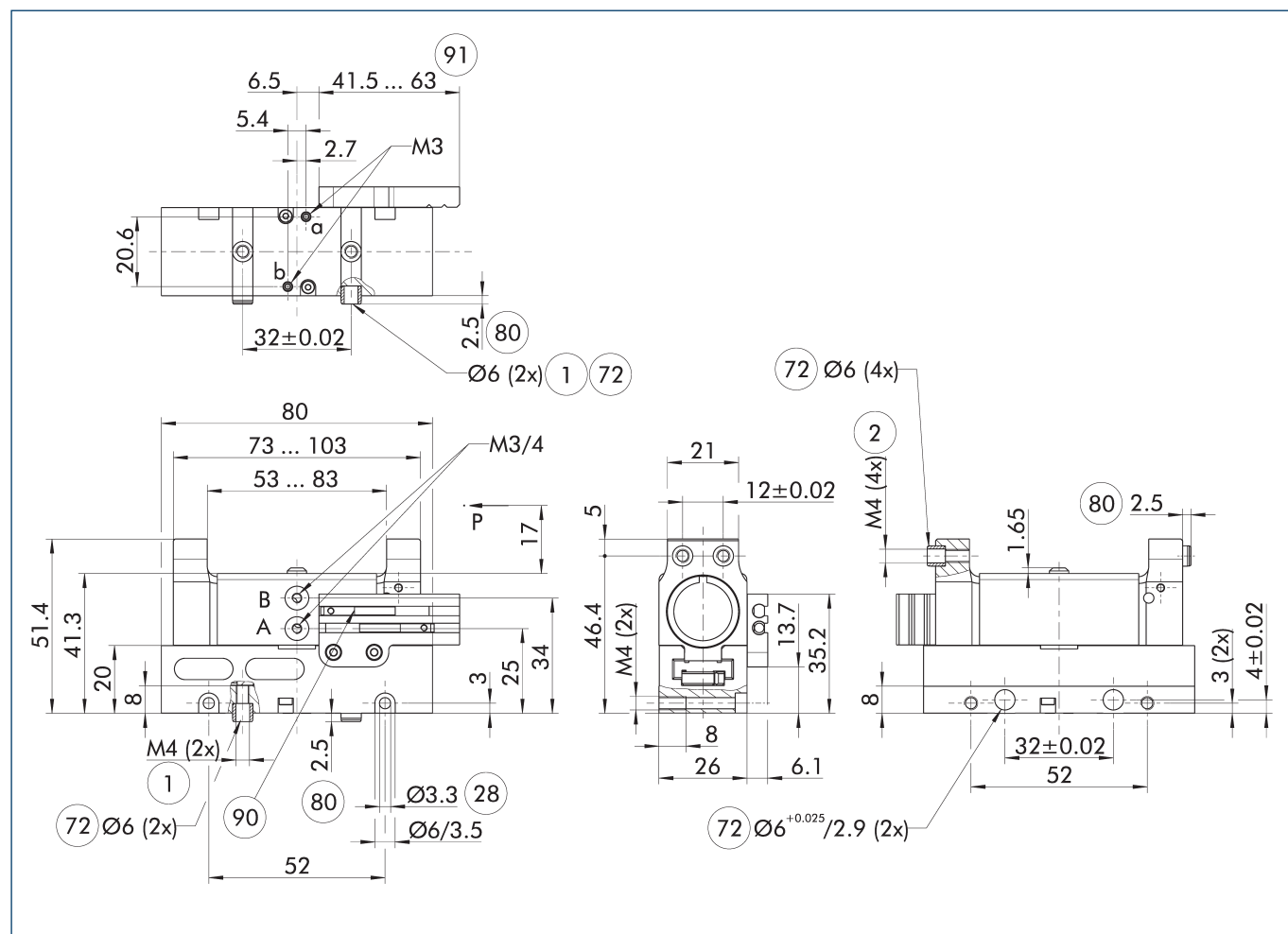
主视图 KGG 80-30
