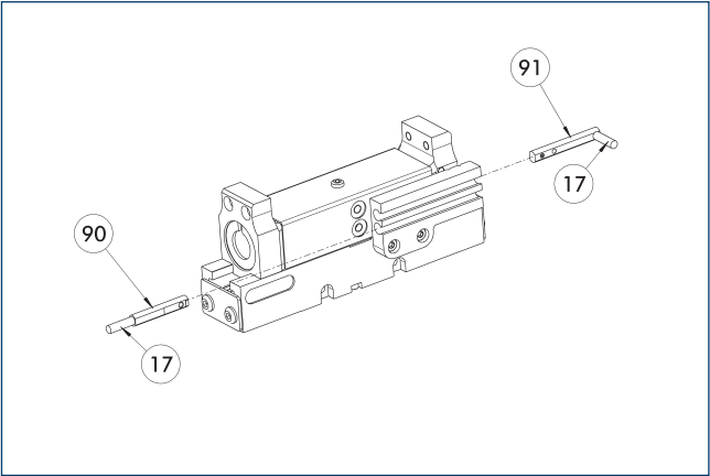
17 电缆出口 91 传感器 MMS 22...-SA 90 传感器 MMS 22..
