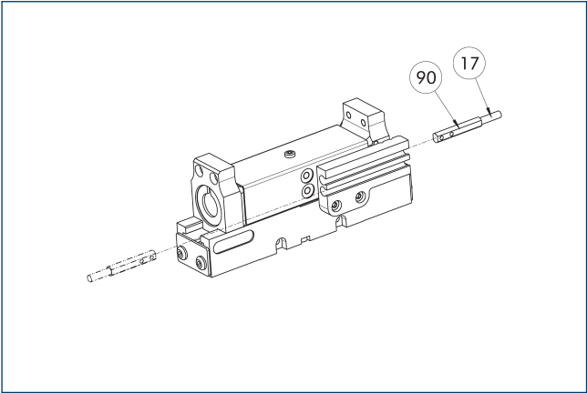
17 电缆出口 90 MMS 22-A-... 传感器 模拟多位置监控，无接触式测量，可用位置数量不限，可轻松安装在 C 型槽中。可以使用 MT 磁性示教工具（在供货范围内，ID 0301030）或 ST 插头式示教工具（选配）编程。用于 C 形槽内安装的终端位置监控。如果表格中列出了 ST 插头式示教工具，则只能使用 ST 示教工具。
