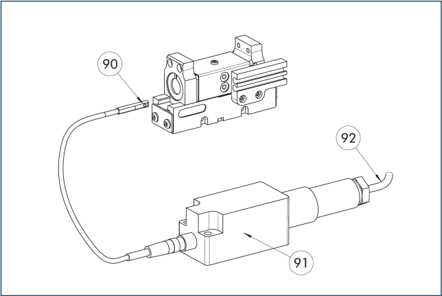
90 MMS 22-A-... 传感器 92 连接电缆 91 FPS-F5电子评价装置
