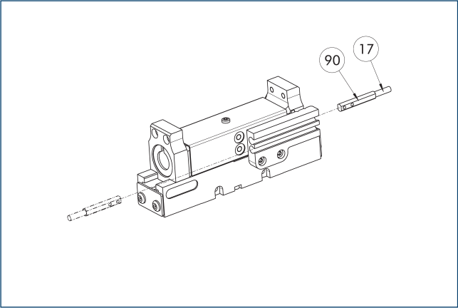
17 Кабельный выход 90 Датчик MMS 22-IO-Link...
