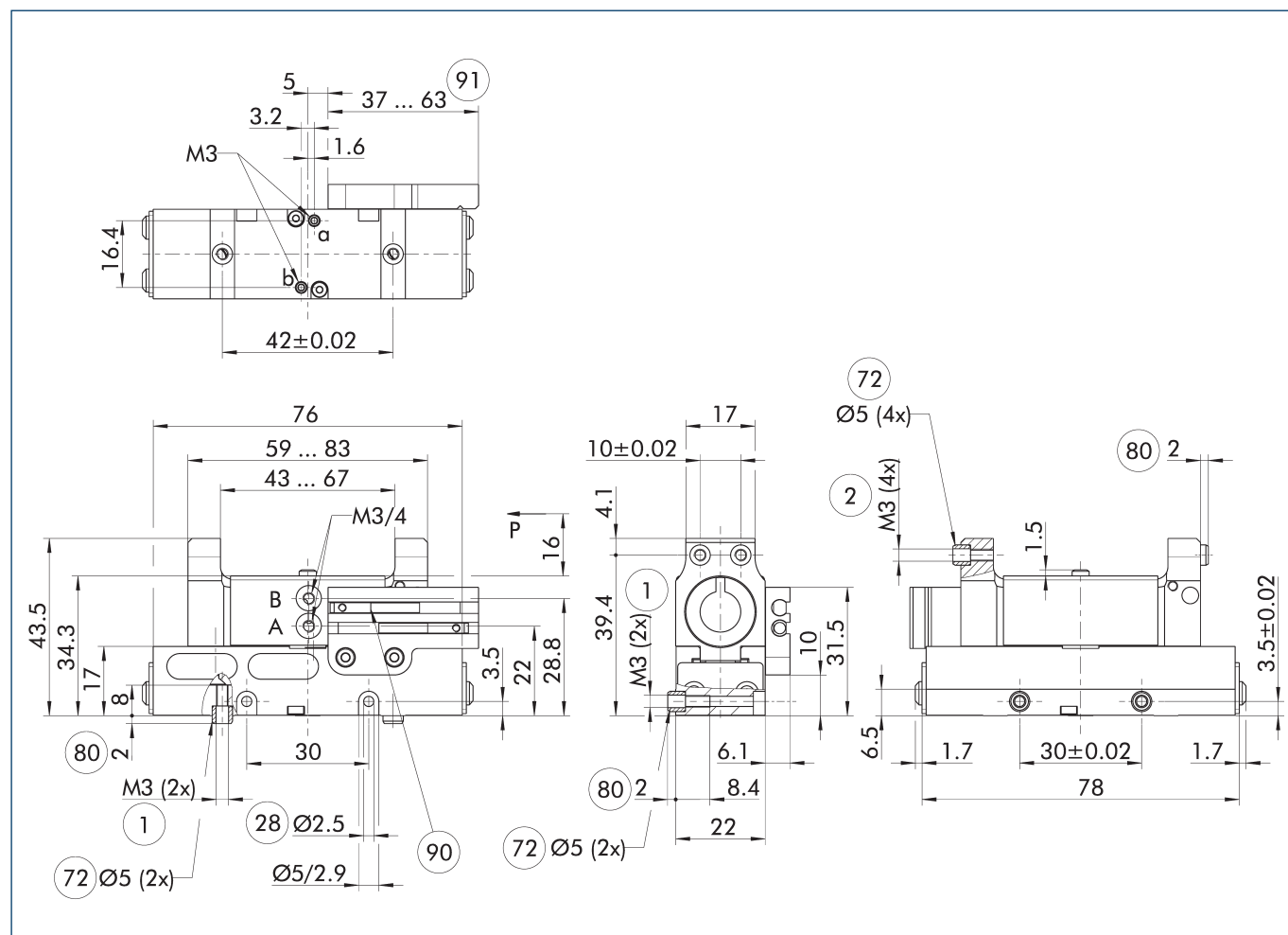
主视图 KGG 70-24
