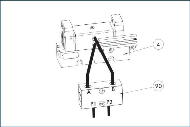
④ 机械手 ⑨⑩ SDV-P 压力保持阀 SDV-P 压力保持阀保证急停期间可临时保持气动夹持、旋转、线性和快换模块的活塞腔压力。
