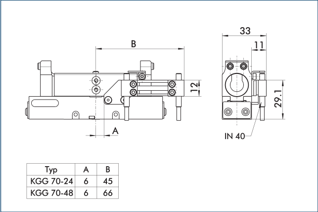
可采用安装套件安装终端位置监控器。 描述 ID 接近式传感器安装套件 AS-KGG 60-20/70-24 0303081 AS-KGG 60-40/70-48 0303080
