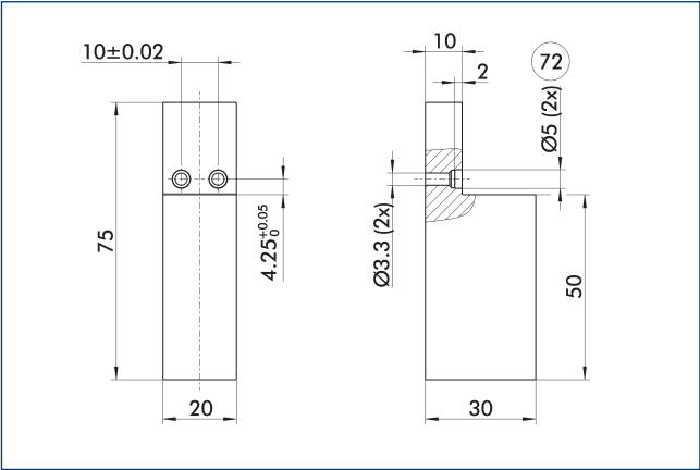
⑦② 适合定心套 该图纸显示了客户可再加工的手指坯件。
