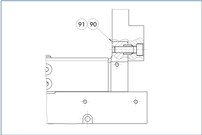
90 Support des doigts de préhension sur le mors de base 91 Voir le plan des doigts ébauches pour les dimensions des doigts de préhension.
