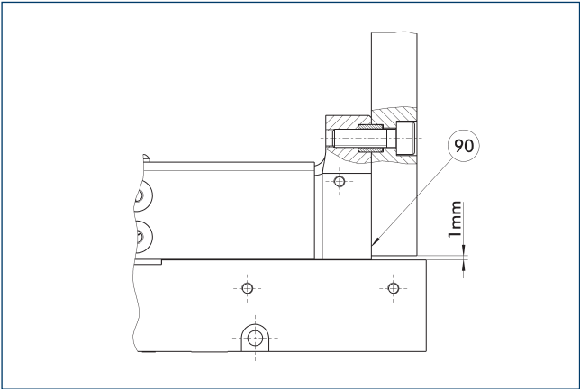
90 Support des doigts de préhension sur le mors de base
