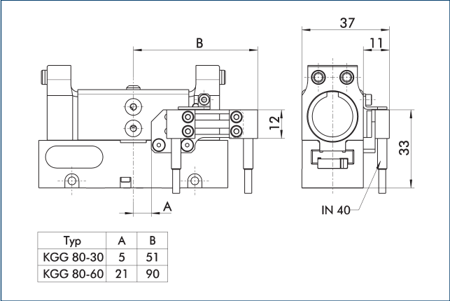
可采用安装套件安装终端位置监控器。 描述 ID 接近式传感器安装套件 AS-KGG 80-30 0303083 AS-KGG 80-60/100-80/140-60 0303084
