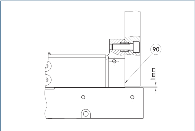
⑨⑩ 在基爪处支撑顶爪
