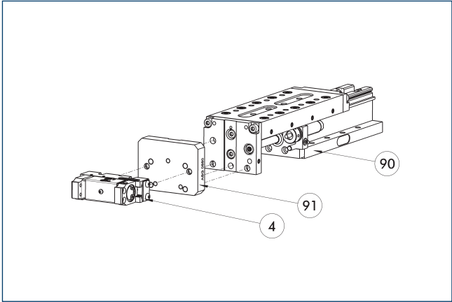
④ Захваты 91 Адаптерная плита ASG 90 Линейный модуль CLM/KLM/LM/ELP/ELM/ELS/HLM
