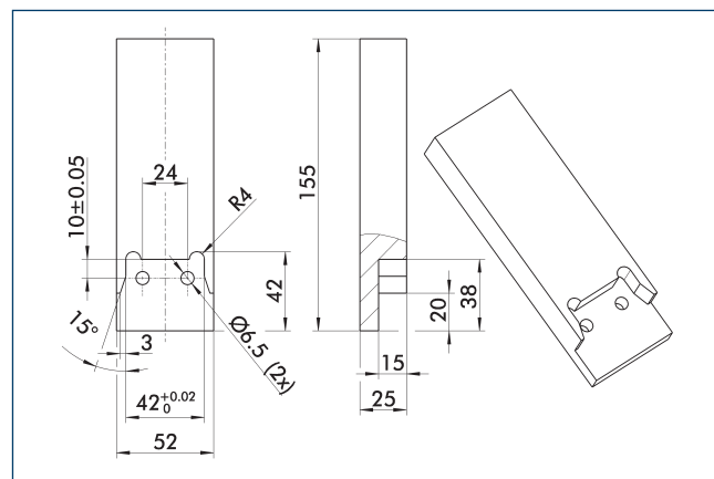
グリッパーフインガーの接続寸法例
