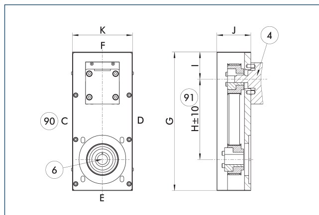
④ Unité linéaire ⑨① Selon le rapport de transmission et la structure de la courroie dentée. ⑥ Raccord d'entraînement ⑨① Renvoi par courroie dans le sens du montage
