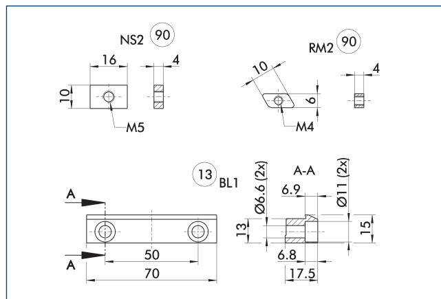
⑬ 安装带
