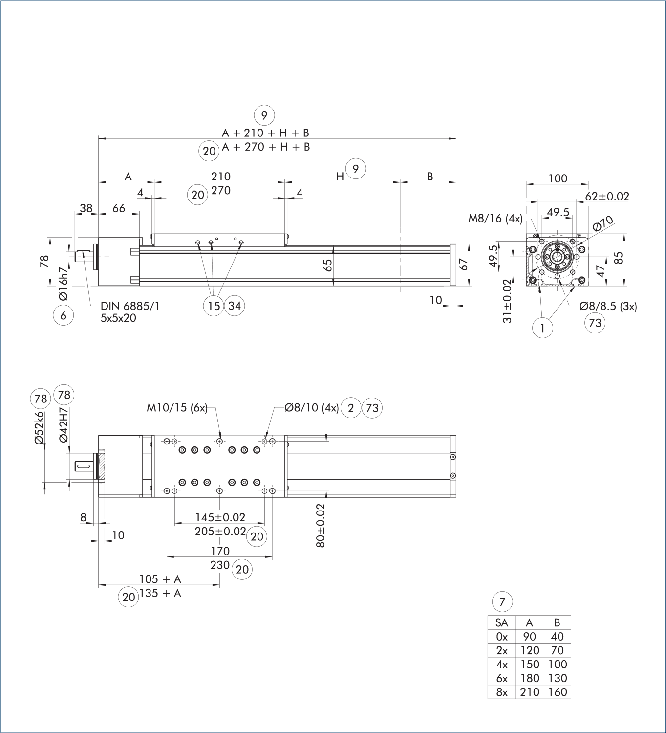
D-SSS 主视图
