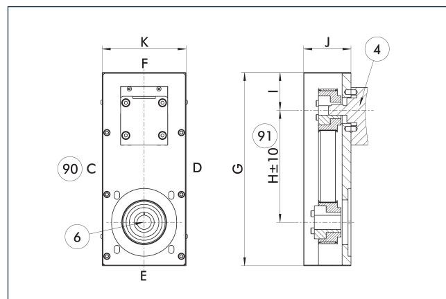
角带传动装置可实现密闭空间的各种传动解决方案。SCHUNK为您的传动装置提供合适的锥齿轮。
