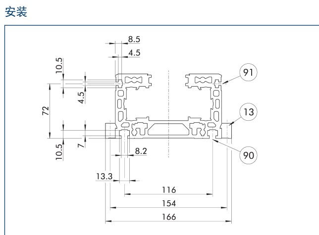
⑬ 安装带 ⑨⑩ 基座侧 T 形螺母 ⑨① 侧向 T 形螺母
