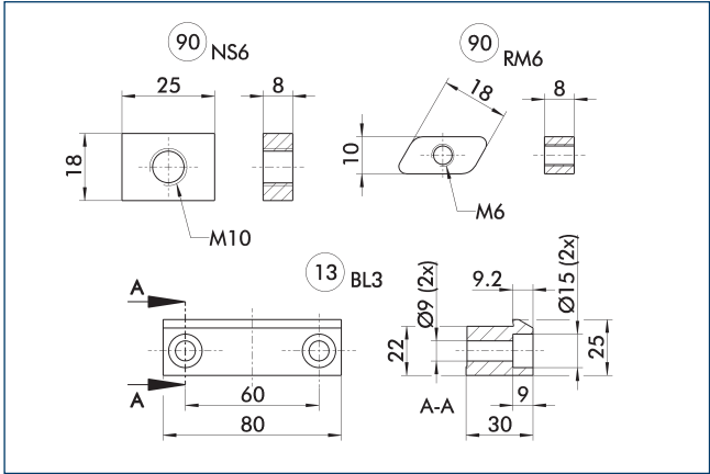
13 安装带
